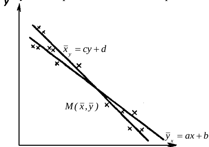
Рис. 4. Лінії регресії x
